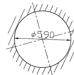
埋込穴寸法
