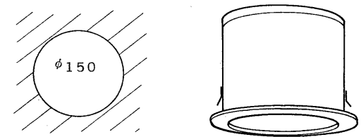
埋込穴寸法
