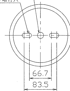
取付寸法図
