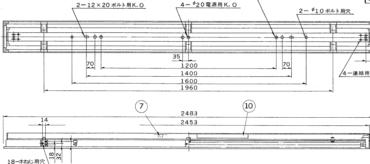
埋込連結使用例
