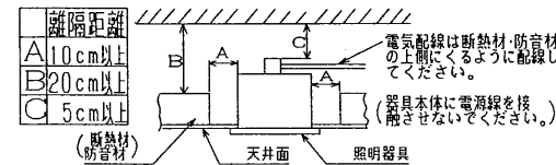
断熱材・防音材をご使用の場合の施工方法
