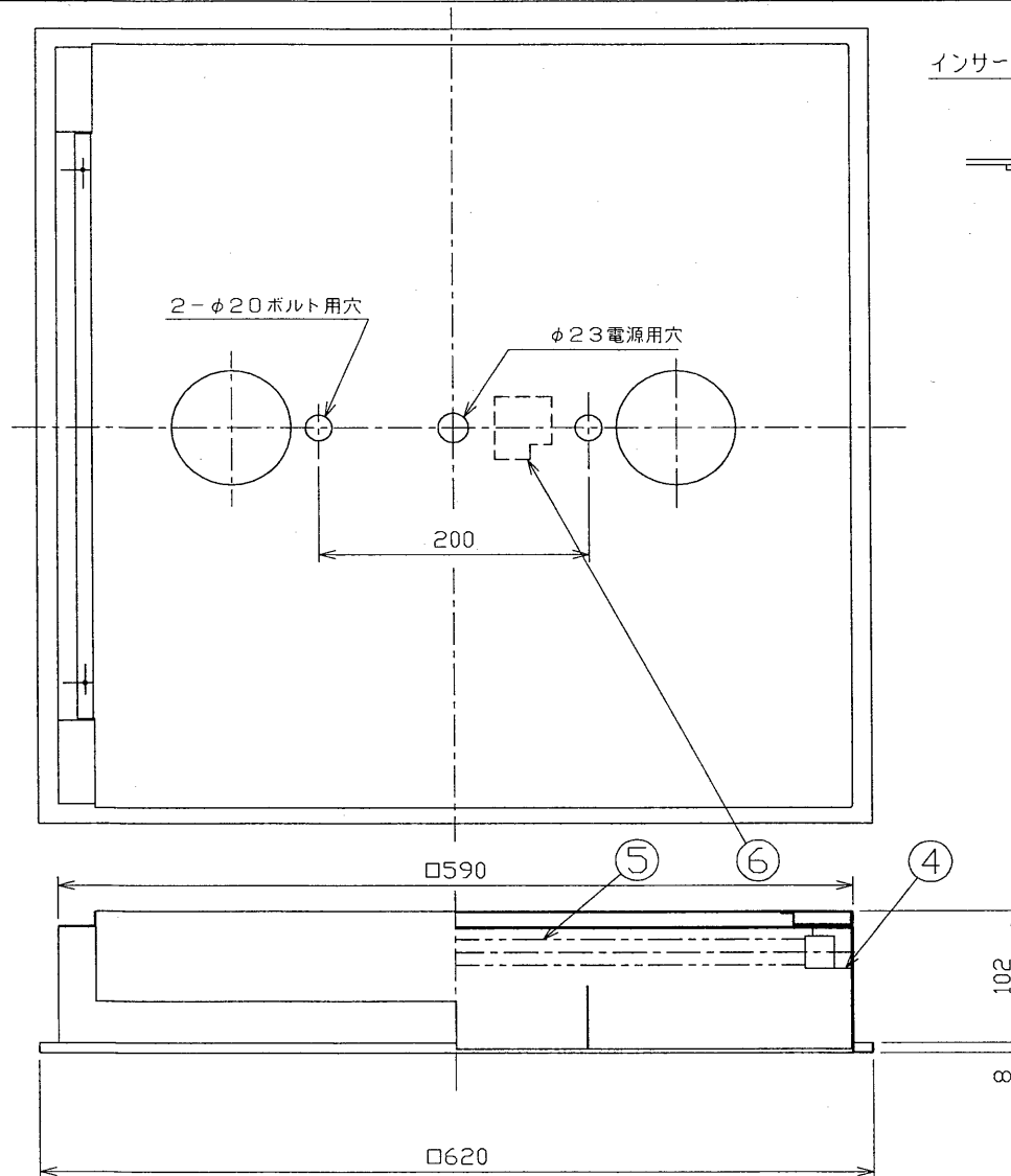
断熱材・防音材をご使用の場合の施工方法
