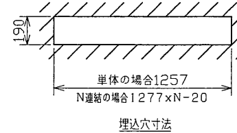
埋込寸法
