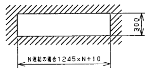
埋込寸法
