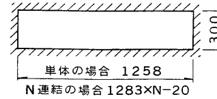
埋込穴寸法
