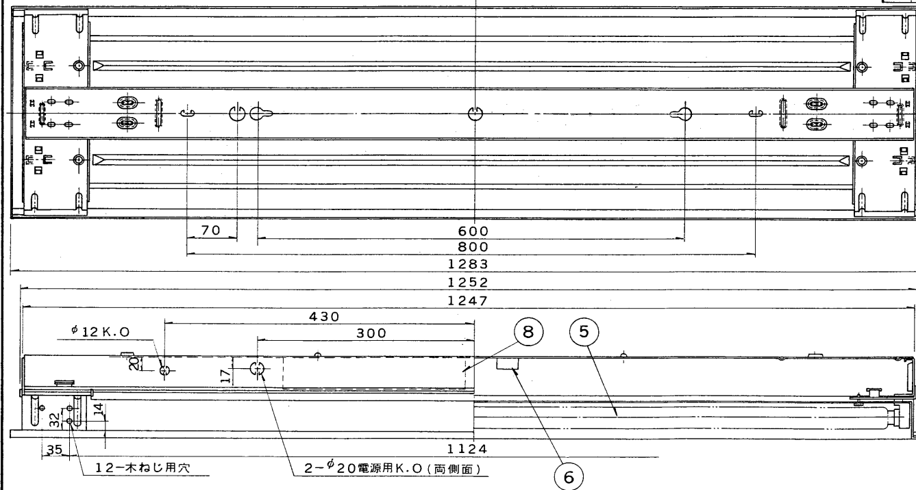
適合連結金具 C-74
