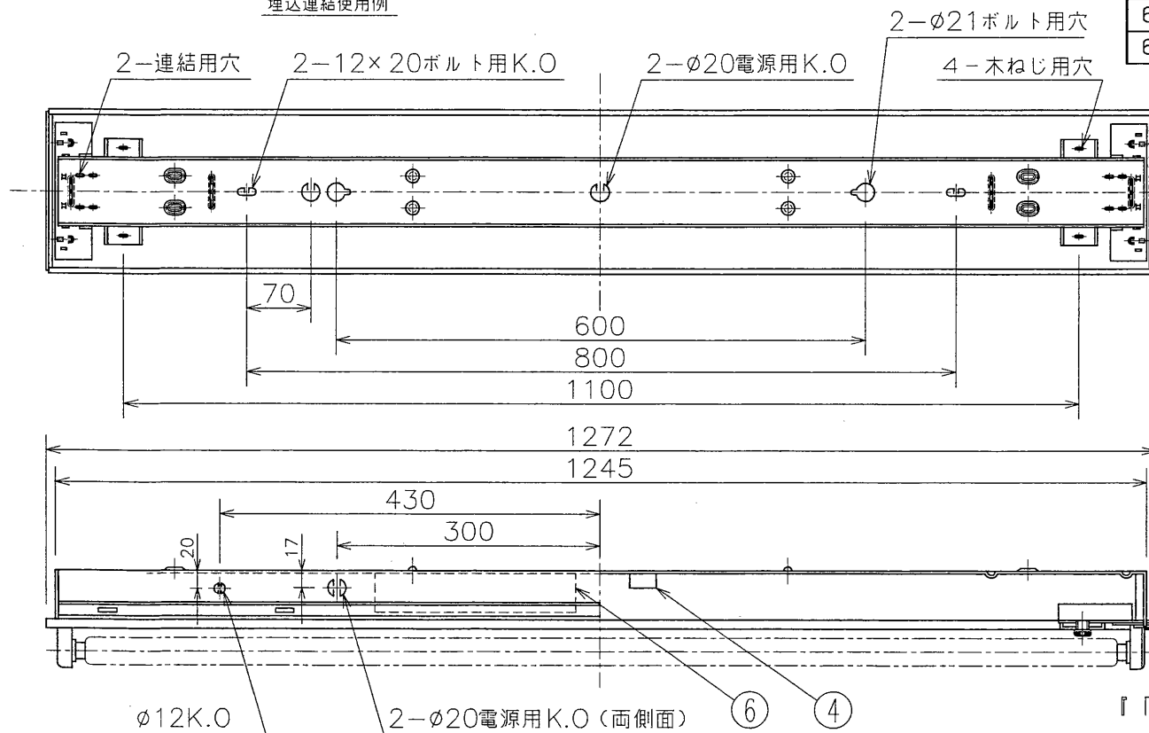
埋込連結使用例
