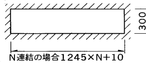
埋込穴寸法
