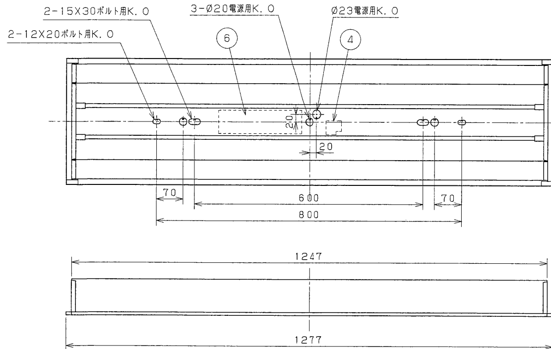
埋込穴寸法
