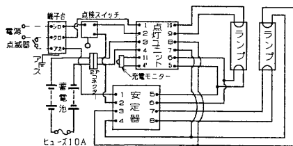
結線圖
