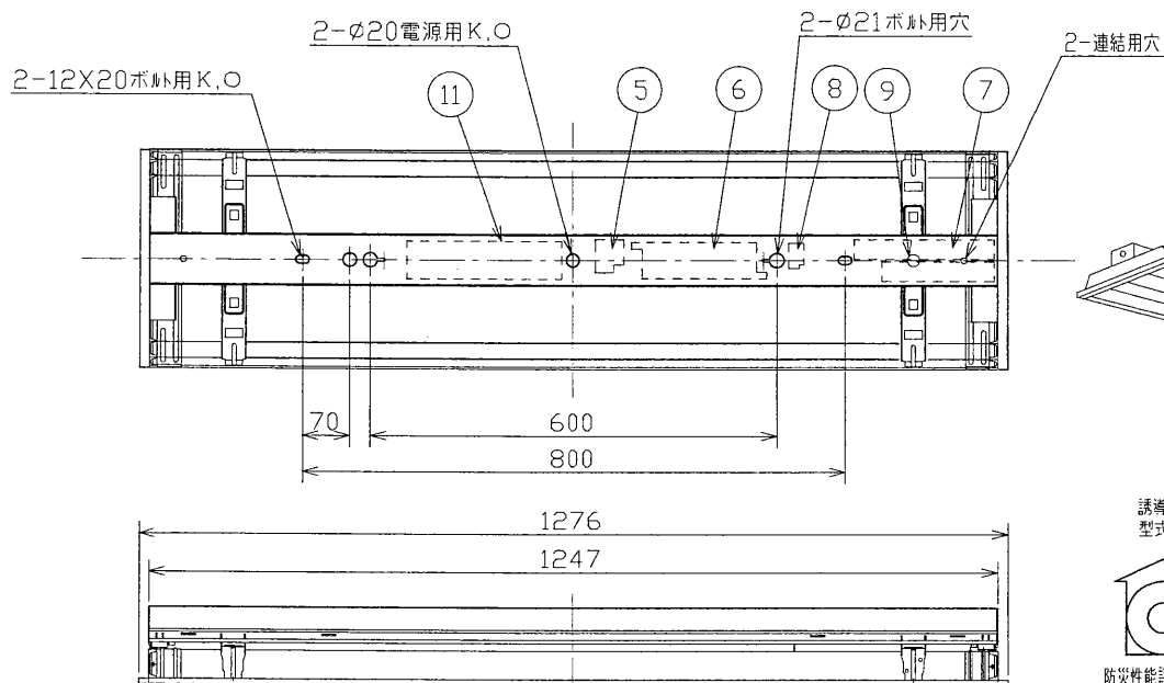
埋込連結使用例
