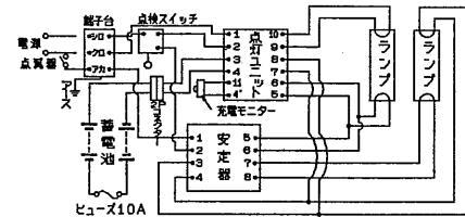
結線図
