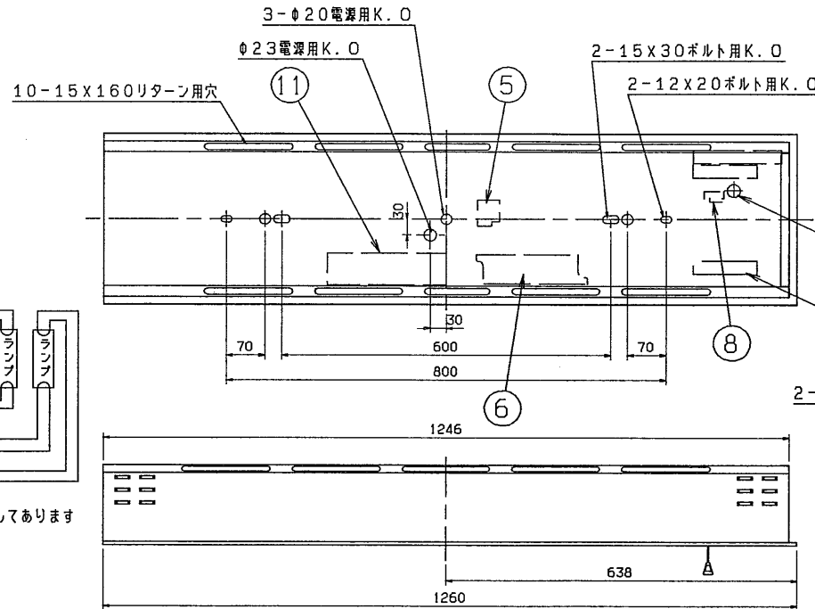
埋込連結使用例
