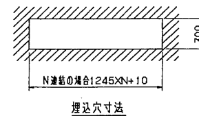
埋込穴寸法
