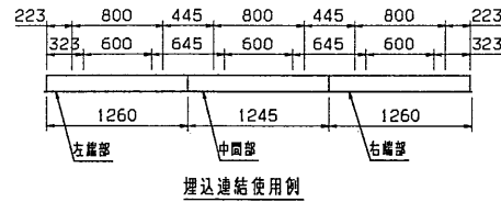
埋込連結使用例
