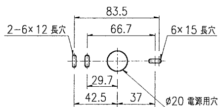
取付寸法図
