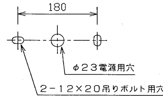
取付寸法図
