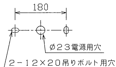
取付寸法図
