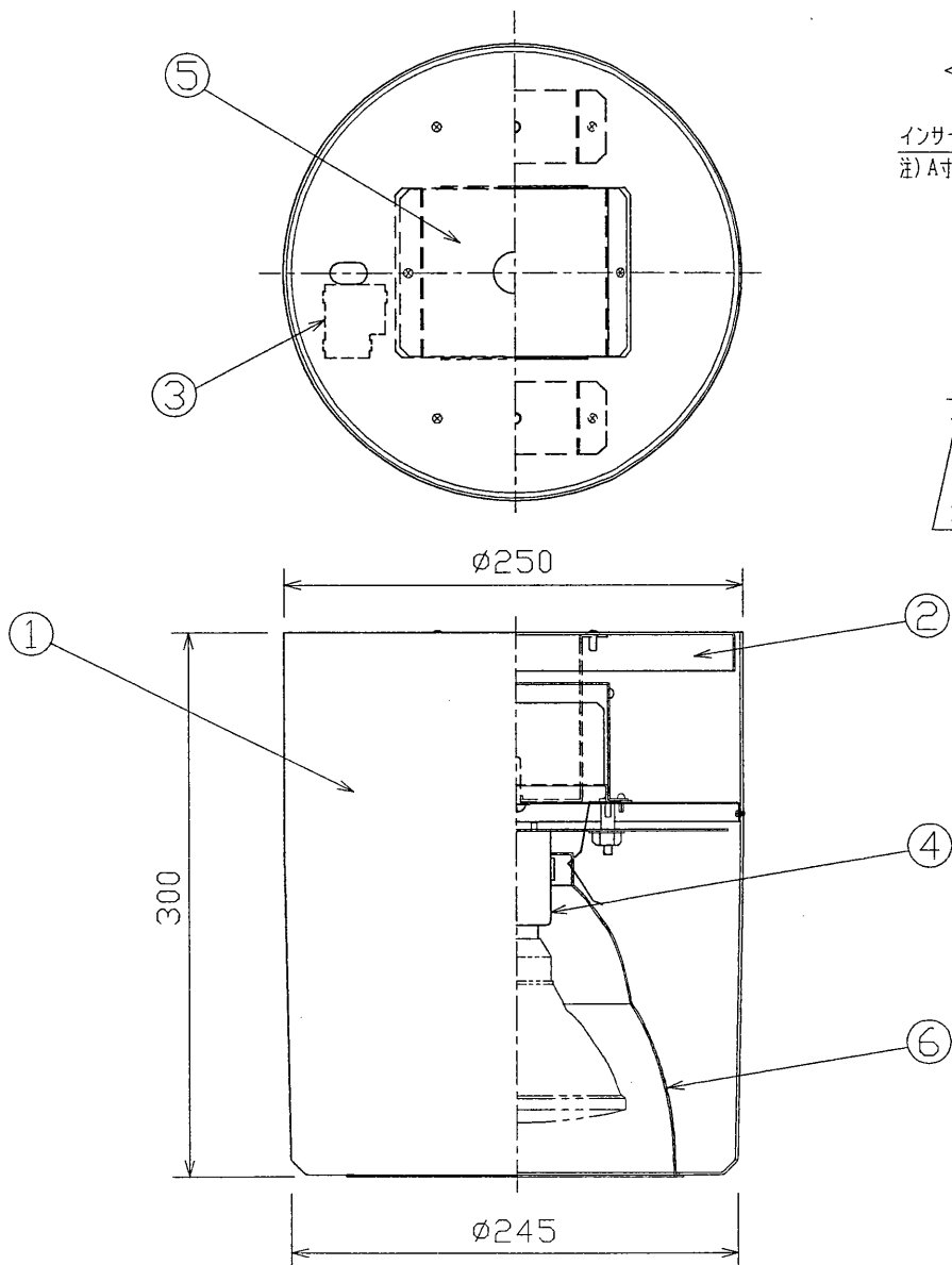
取付寸法図
