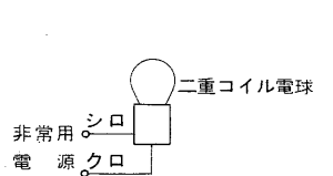
結線図(非常灯回路のみ)
