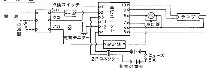
結線図
