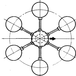
6 灯 用 60°等間隔
