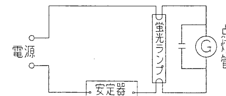
結線図
