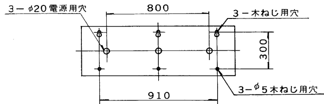
取付寸法図
