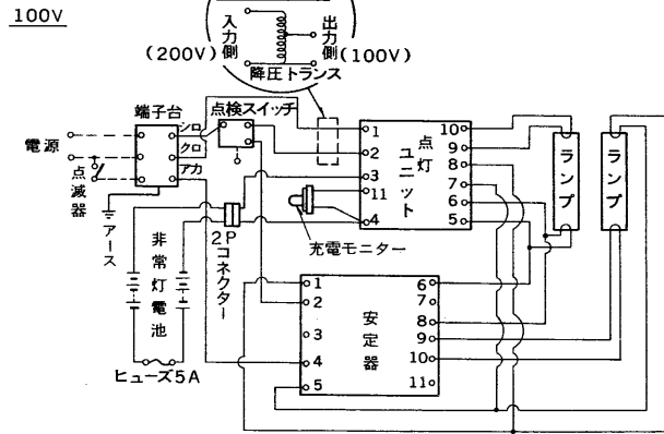
結線図
