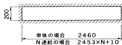
埋込穴寸法
