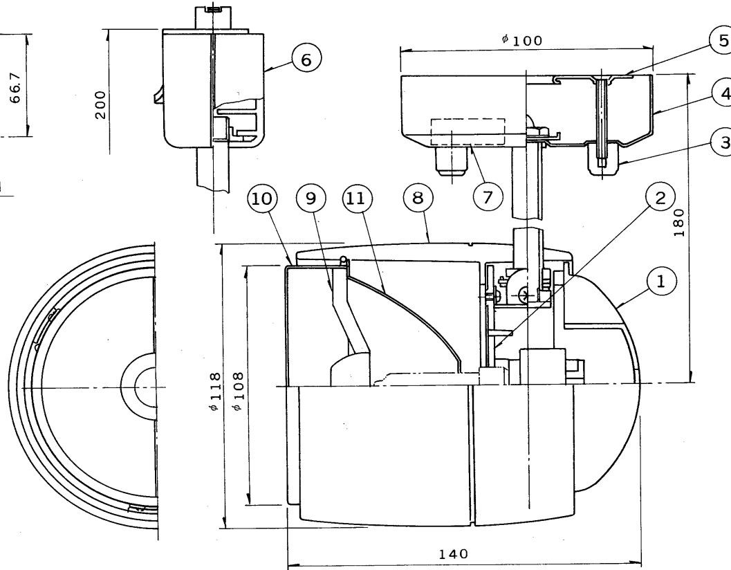
取付寸法図
