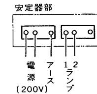
結 線 図
