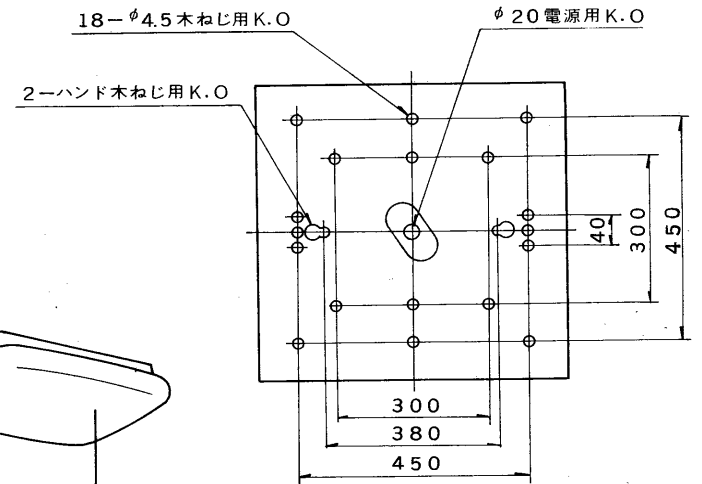
取付寸法図
