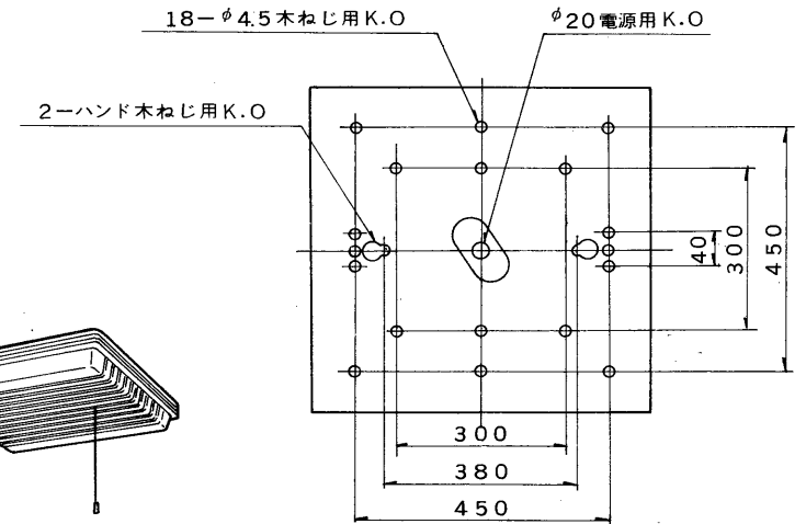
取付寸法図 防虫形
