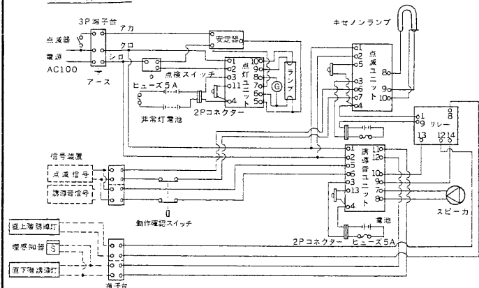
結 線 図
