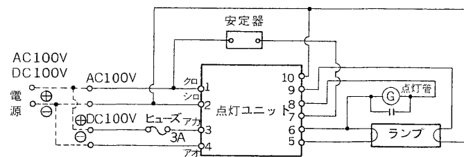
結 線 図
