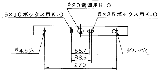
壁面取付用
