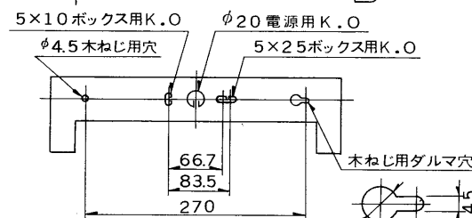
棚下取付用
