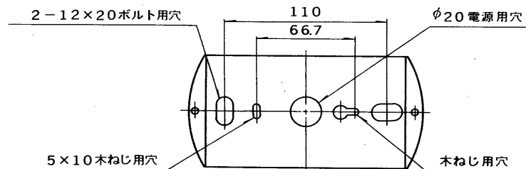
取付寸法図
