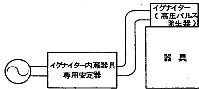
配線図
