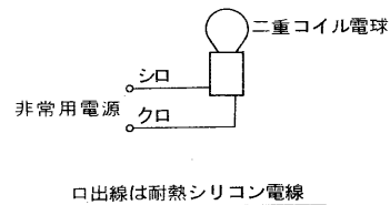
結 線 図
