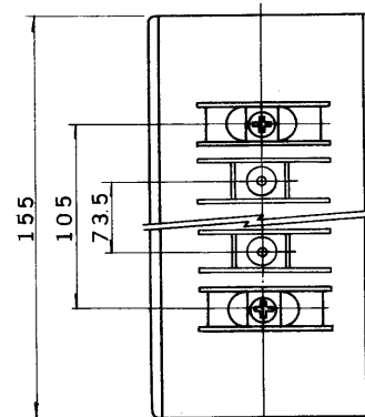
SK-23 (連結用)
