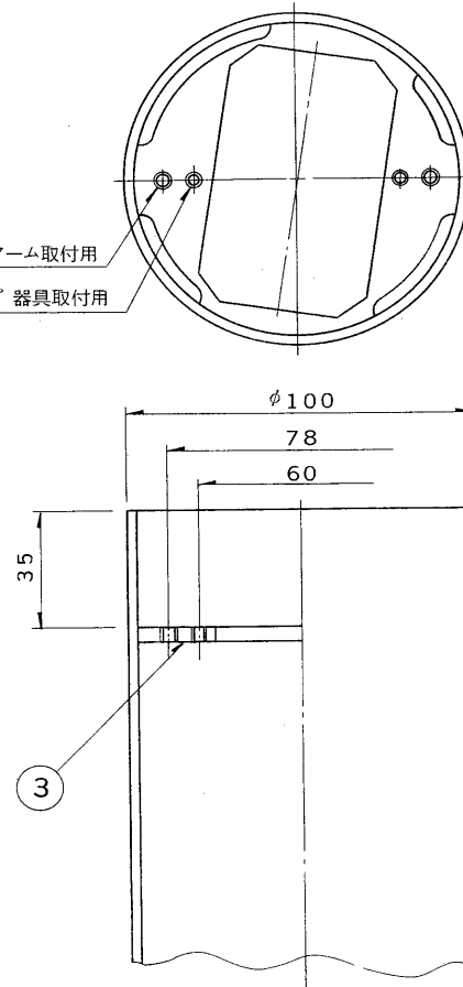
ポール先端部詳細図
