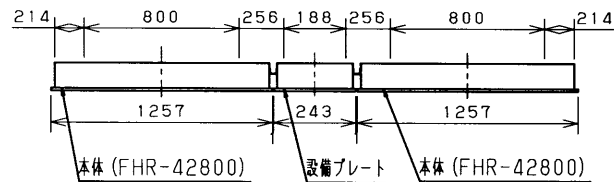
埋込連結使用例
