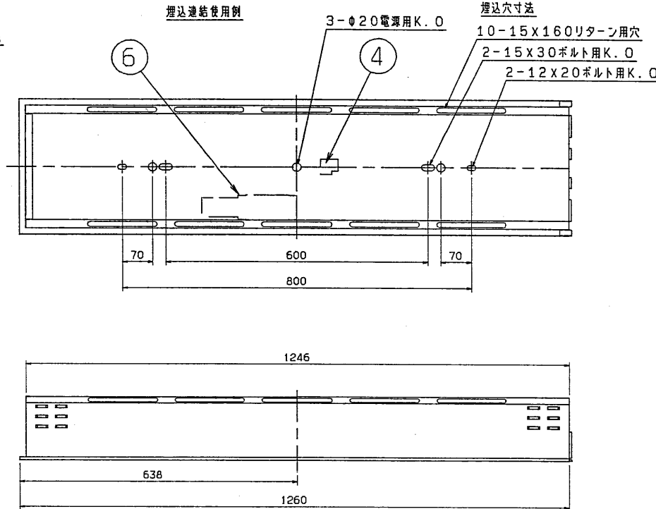
インサートボルトの器具内寸法
