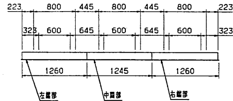
埋込連結使用例
