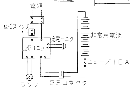
結線図
