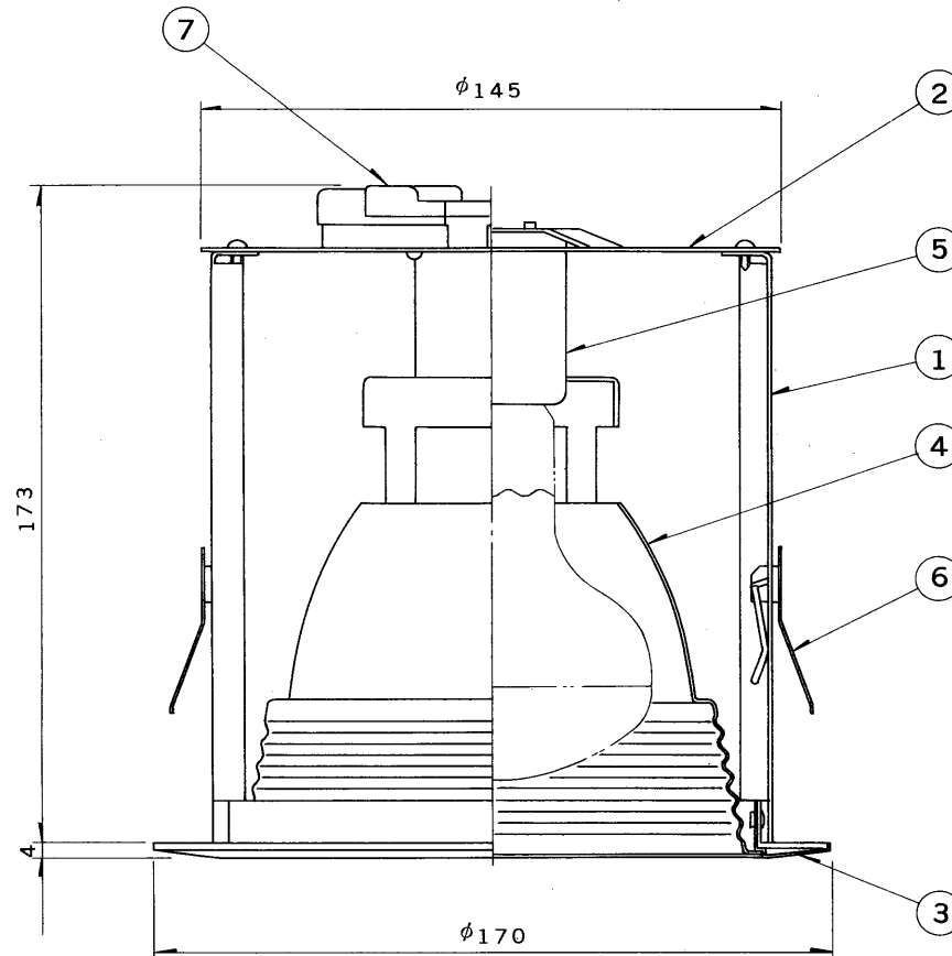
埋込穴寸法 天井取付厚さ：3～40mm
