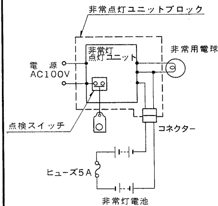
結線図
