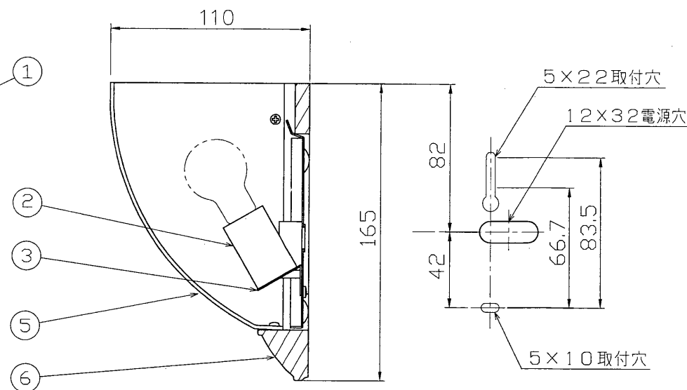
取付寸法詳細正面図
