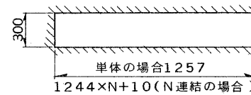
埋込穴寸法
