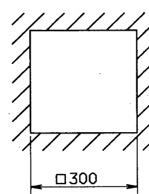
埋込穴寸法
