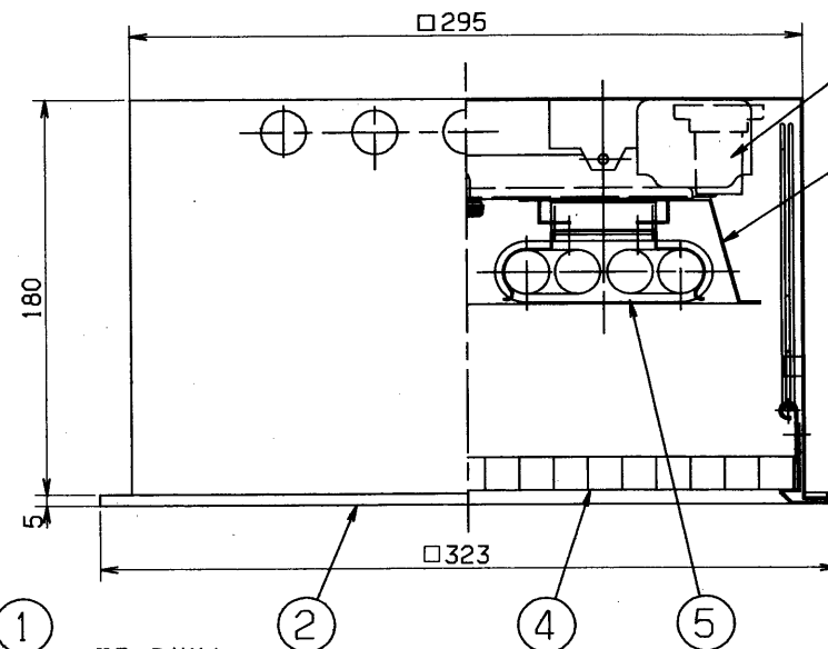
埋込穴寸法
