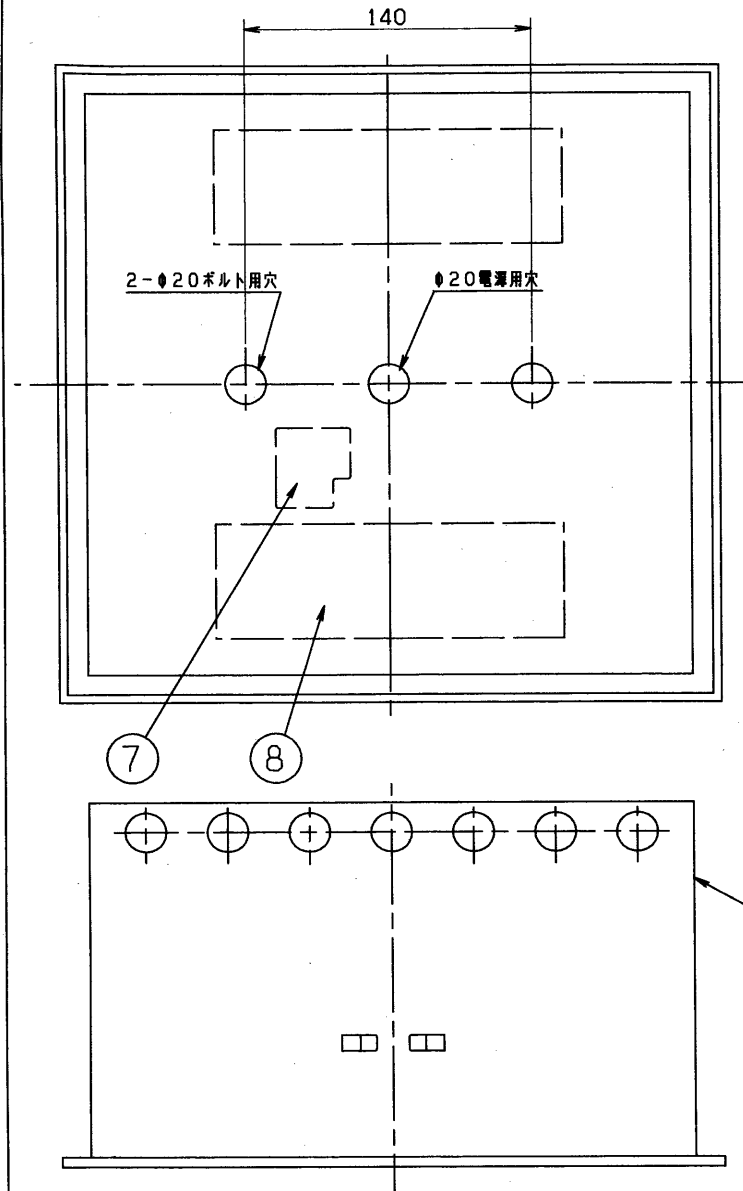
埋込穴寸法
