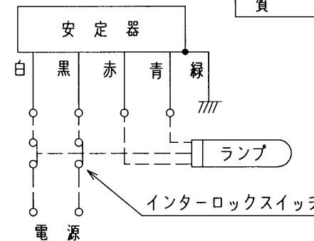
結線図
