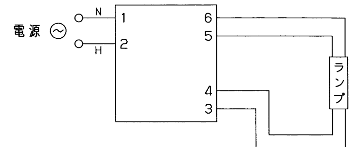
結線図
