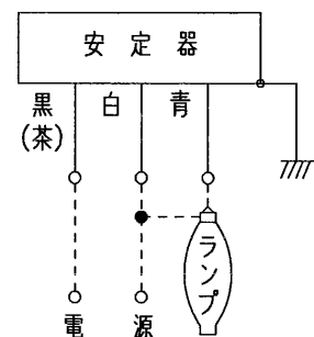
結線図
