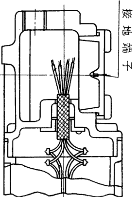
端子箱断面
