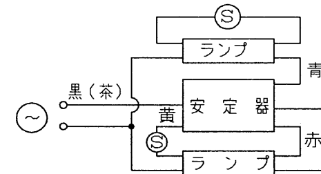
結 線 図
