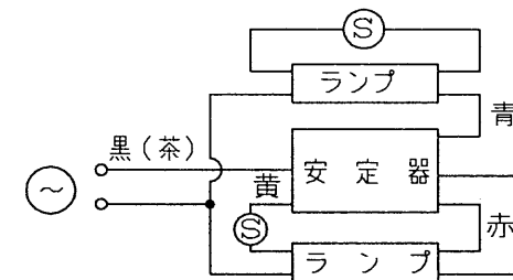
結 線 図
