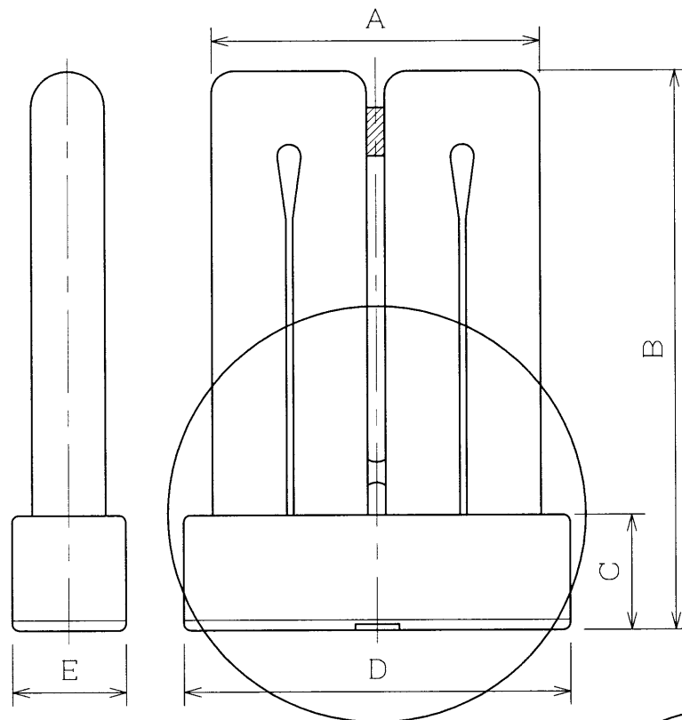
裏面口金ピン部拡大図
